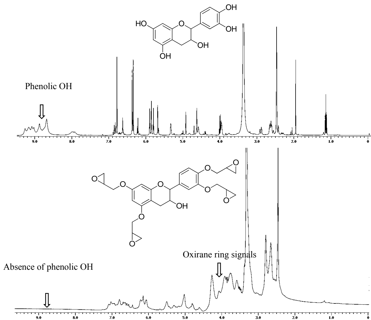
Figure 7: The ^1\text{H} NMR of HDGTE and GEHDGTE.
